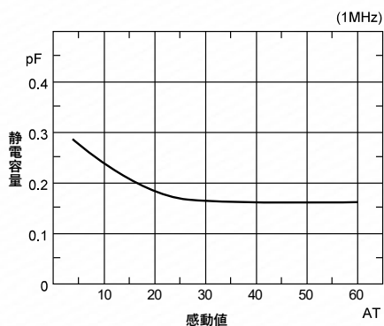
接点間静電容量
